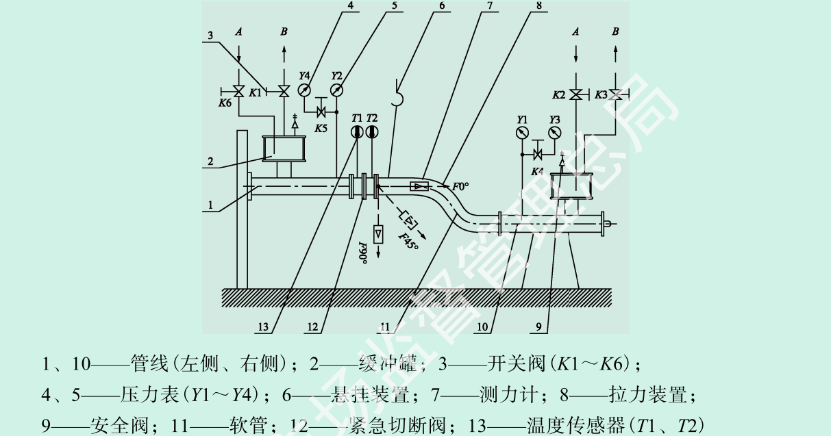
图 G-1 致断螺栓切断阀拉断性能试验装置
