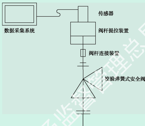
图 dc-5 在线校验辅助开启装置
