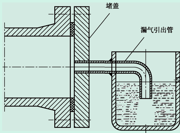
图 dc-3 气泡计数检漏装置
