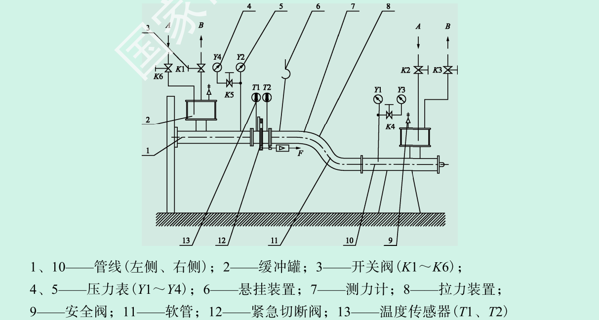
图 G-2 拉索断开切断阀拉断性能试验装置
