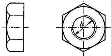
图 3.0.5-1 I型及II型六角螺母(示例)
